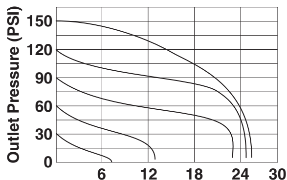
Fig. 3 Valve 40-881-19
