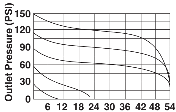
Fig. 4 Valve 40-882-17
