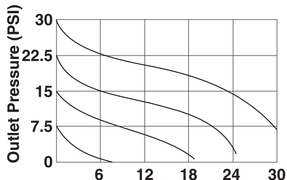
Fig. 3 Valve 40-881-19
