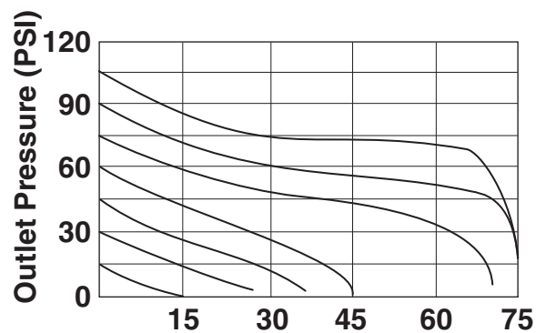
Fig. 8 Valve 40-883-11
