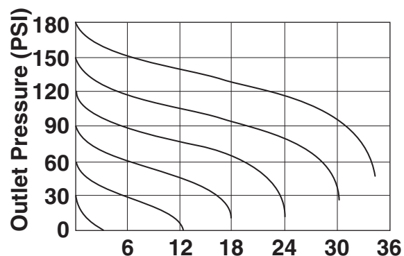
Fig. 4 Valve 40-882-17
